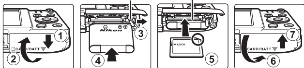
Batterijvergrendeling Geheugenkaartsleuf
